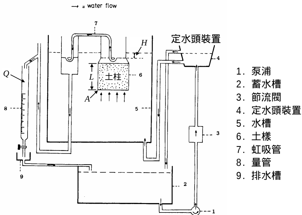
圖 3. 水力傳導度儀器運作原理
