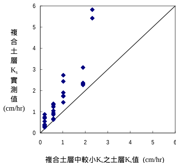
圖 5. 雙層複合土層與其土層中較小飽和水力傳導度之比較
