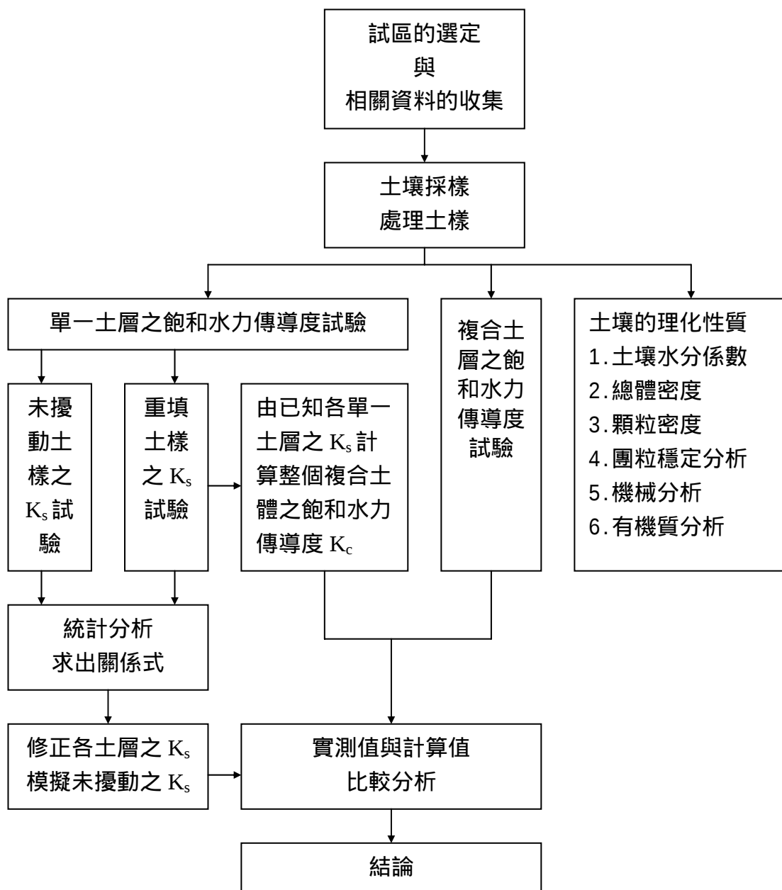
圖 2. 研究流程圖
