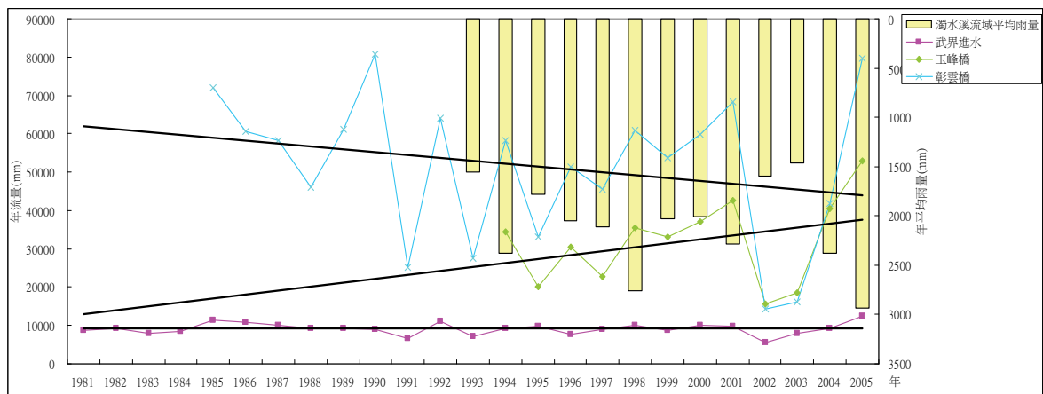
圖 8 濁水溪流域流量變化趨勢圖
