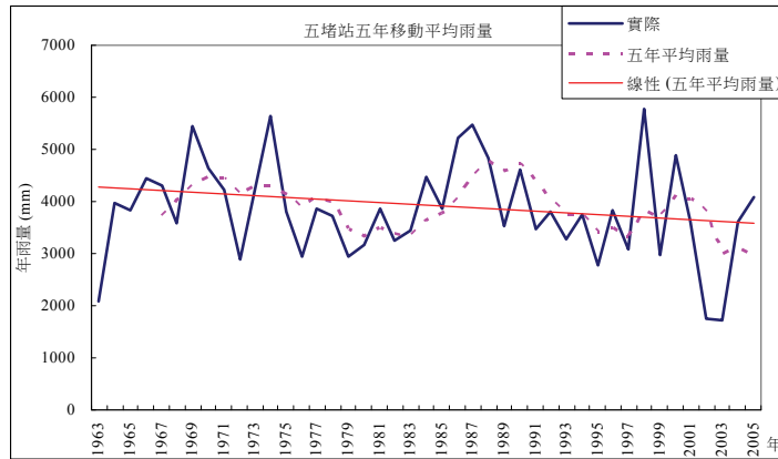
圖 10 五堵站五年移動平均雨量變化趨勢圖
