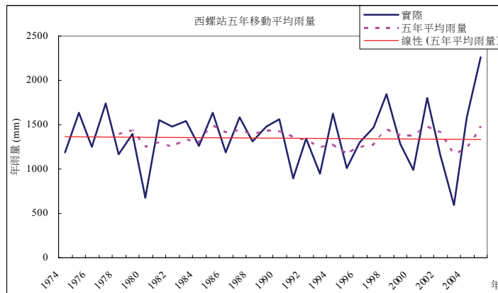
圖 14 西螺站五年移動平均雨量變化趨勢圖
