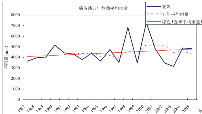
圖 9 瑞芳站五年移動平均雨量變化趨勢圖
