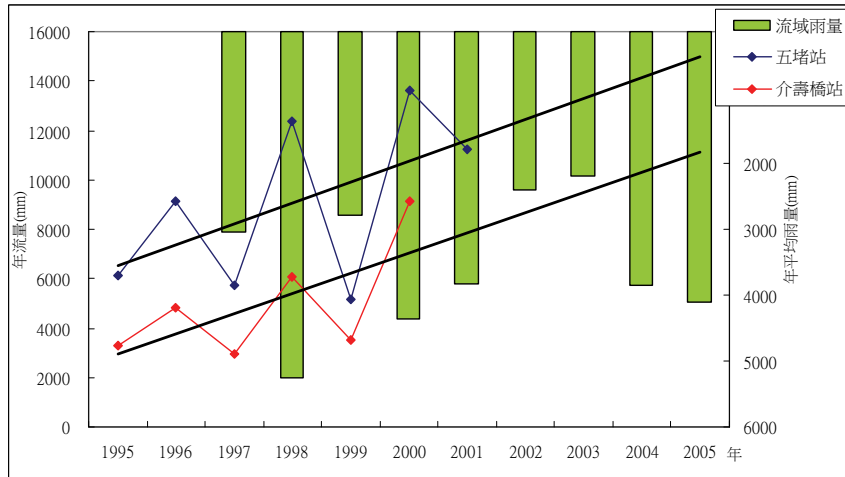
圖 7 基隆河流域流量變化趨勢圖
