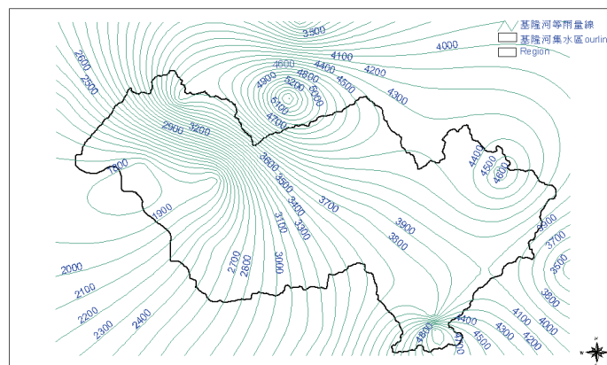
圖 2 基隆河流域等雨量分佈圖
