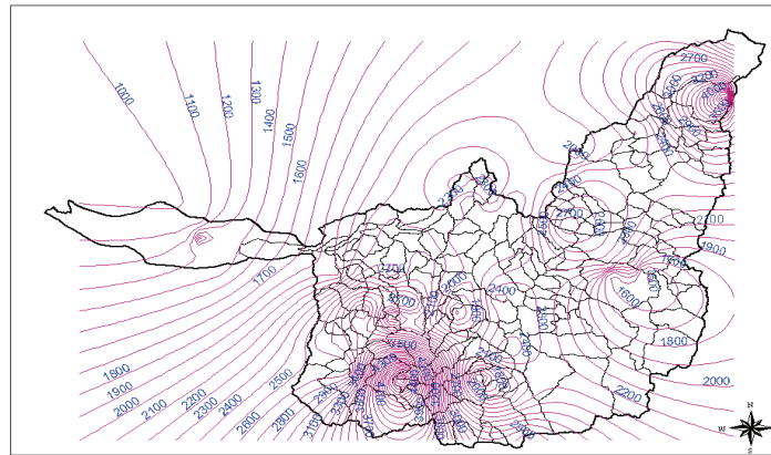
圖 3 濁水溪流流域等雨量分佈圖
