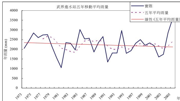
圖 12 武界進水站五年移動平均雨量變化趨勢圖
