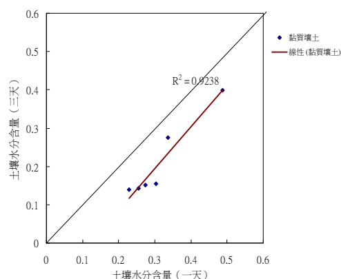
圖 9. 粘質壤土水分含量線性迴歸分析
