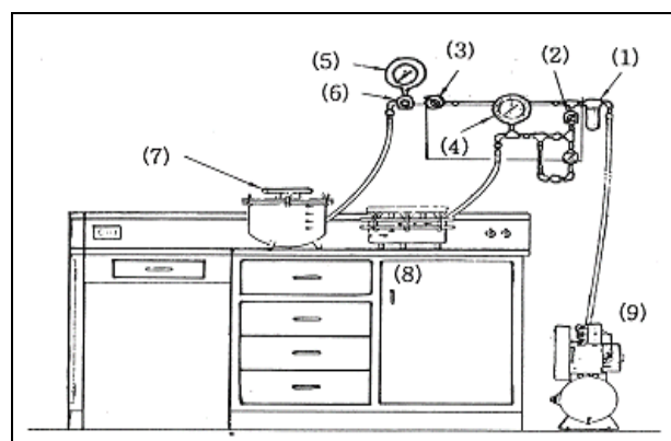
圖 3. 壓力鍋實驗裝置
