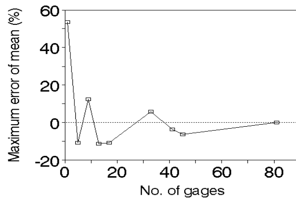
圖 5. 天然闊葉林 12 場不同數量量筒穿落雨的最大誤差率
