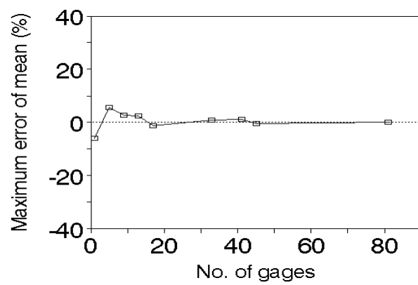
圖 7. 空曠地 12 場不同數量量筒降雨的最大誤差率
