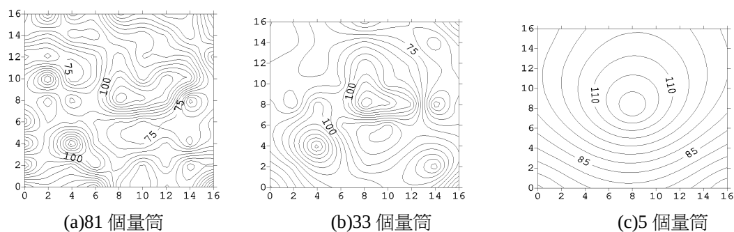
圖 8. 天然闊葉林不同數量量筒 ((a)81 個量筒(b)33 個量筒(c)5 個量筒) 量測穿落雨的空間分佈特性(20 公分直徑承雨口，穿落雨 86.8mm，1997,6,5)
